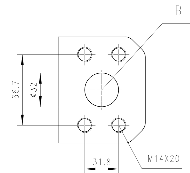
Y向视图
